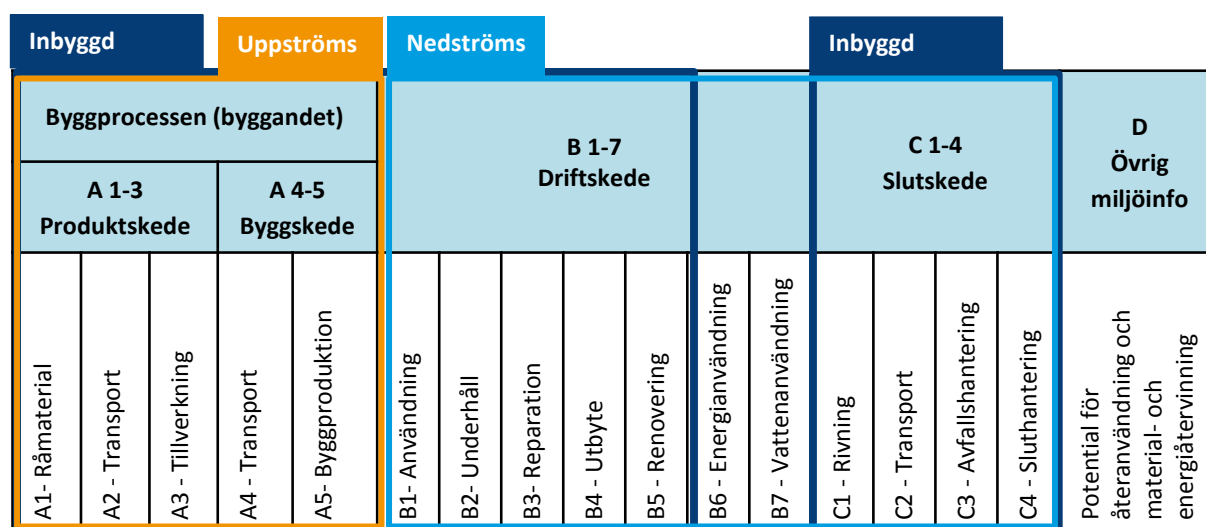
Figur 4: Illustration av begreppen uppströms, nedströms och inbyggd så som de definierats i detta projekt.
