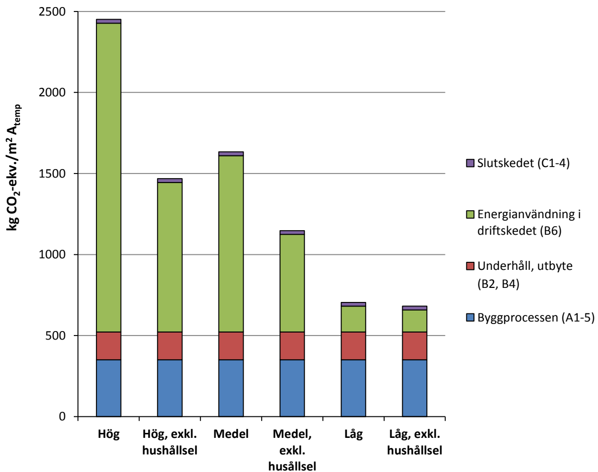
Figur 16: Fördelning av klimatpåverkan över livscykeln vid en analysperiod på 100 år.
