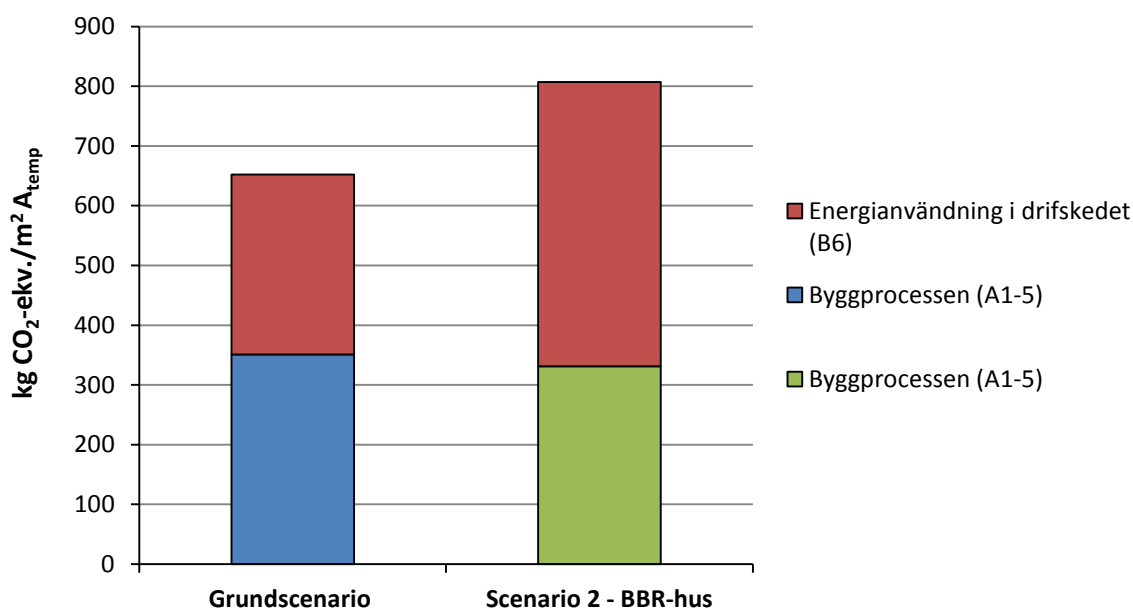
Figur 20: Fördelning av total klimatpåverkan mellan modulerna A1-5 och B6 – jämförelse mellan grundscenariot och ett hus konstruerat för att uppfylla kraven i BBR. Analysperioden är 50 år.
