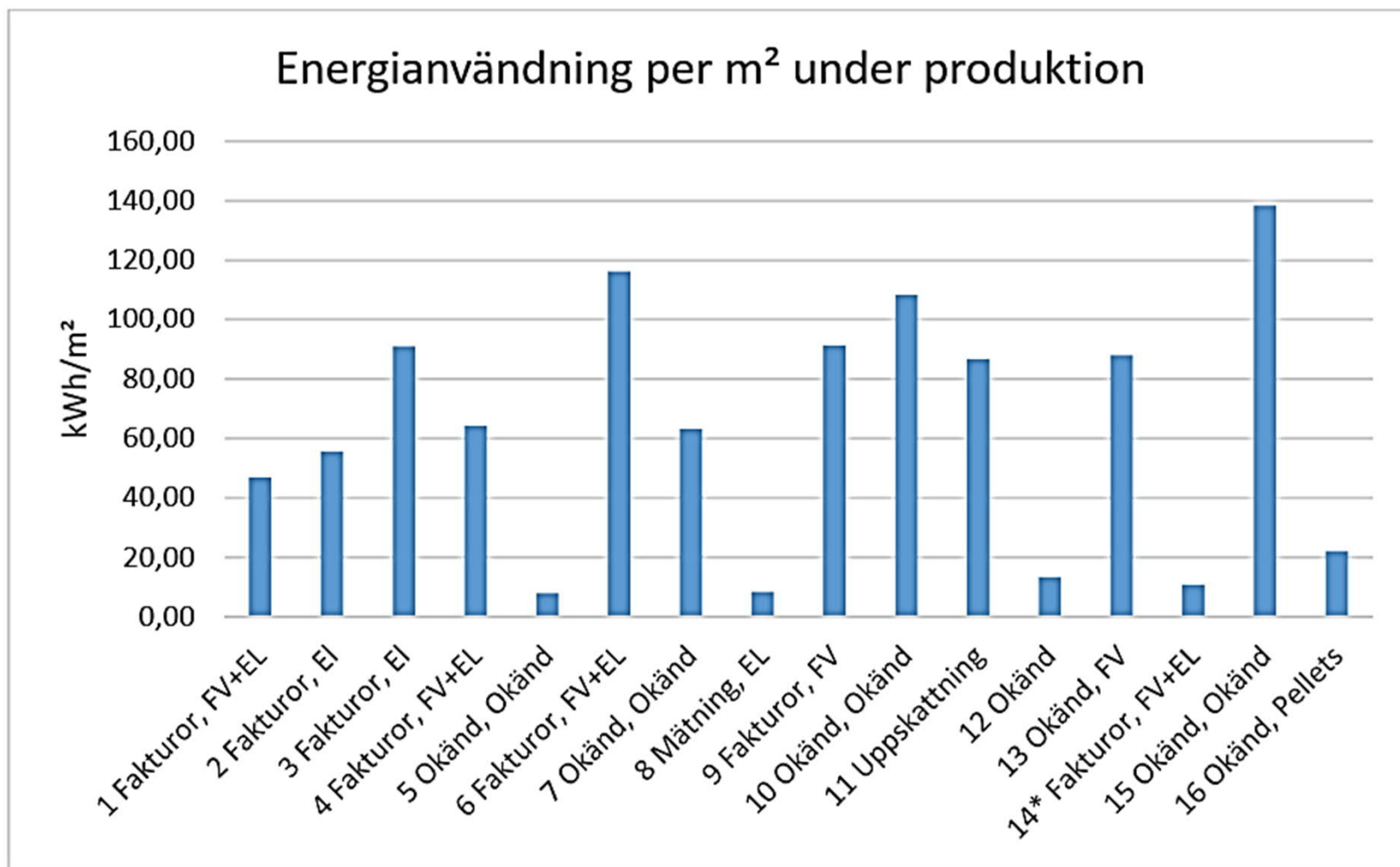
Figur 18 Energianvändning per m 2 under produktion
