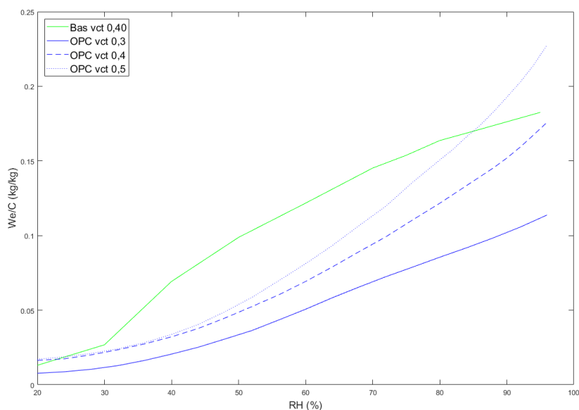
Figur 3. Jämförelse av desorptionskurvor, bunden fuktmängd per cementmängd (kg vatten per kg cement) som funktion av relativ fuktighet (%). OPC - källa: Betonghandboken, Nilsson 1980. Bascement – källa: opublicerad, pågående inmätning av Stelmarczyk et al. 2018 inom SBUF Projekt 13198 samt 13140.
