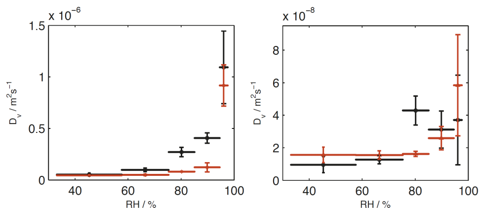
Figur 4. Jämförelse av transportkoefficient för ånghalt som funktion av relativ fuktighet. Till vänster – CEM I (OPC) vct 0.4, till höger – CEM III B (30% klinker + 70% slagg) vct 0.4, svart – under desorption, röd – under absorption. Källa: Saeidpour, Doctoral Thesis, Paper III, LTH 2015.
