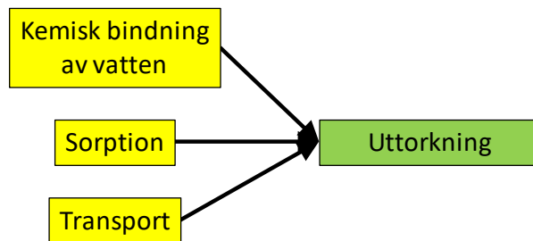
Figur 1. Förenklad bild av fenomenet bakom uttorkning av betong.
