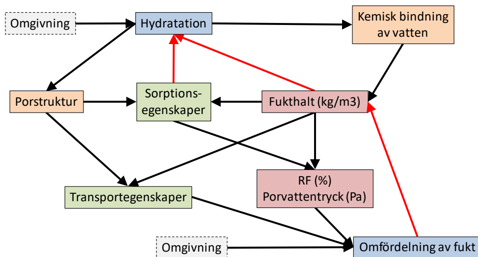
Figur 2. Fenomen och inbördes beroenden under uttorkning av betong.
