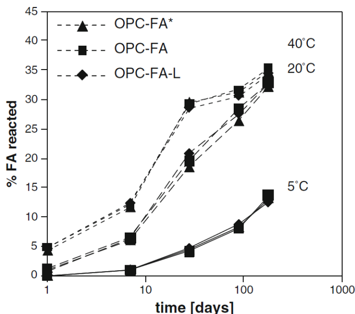
Figur 4. Reaktionsgrad för flygaska som funktion av tid vid olika temperaturer, OPC-FA*: 70% OPC +30% FA, OPC-FA: 65% OPC + 35% FA, OPC-FA-L: 65% OPC + 30% FA + 5% kalkstensfiller, från De Weerd m.fl. 2012.
