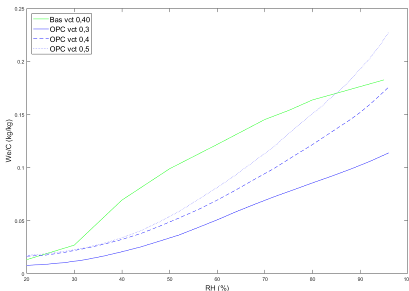
Figur 9. Fuktalt We/C som funktion av relativ fuktighet vid desorption för betong med Bascement (från Stelmarczyk m.fl. 2017b) resp. OPC (från Nilsson 1980).
