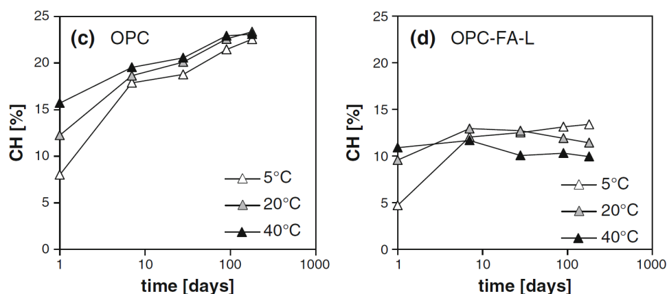
Figur 5. Mängd bildad portlandit (förhållande till totalvikten av bruk utan vatten) som funktion av tid vid olika temperaturer, OPC: 100% OPC, OPC-FA-L: 65% OPC + 30% FA + 5% kalkstensfiller, från De Weerd m.fl. 2012.
