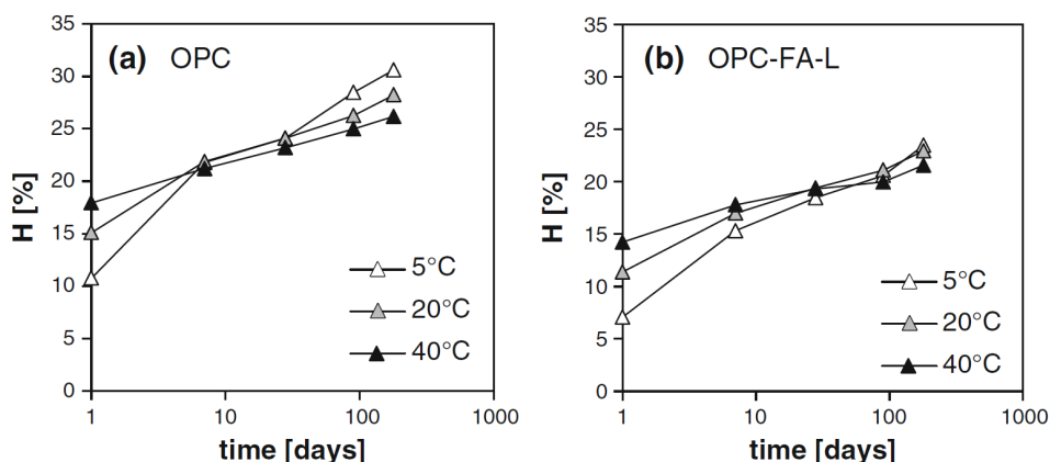
Figur 6. Mängd kemiskt bundet vatten (förhållande till totalvikten av bruk utan vatten) som funktion av tid vid olika temperaturer, OPC: 100% OPC, OPC-FA-L: 65% OPC + 30% FA + 5% kalkstensfiller, från De Weerd m.fl. 2012.
