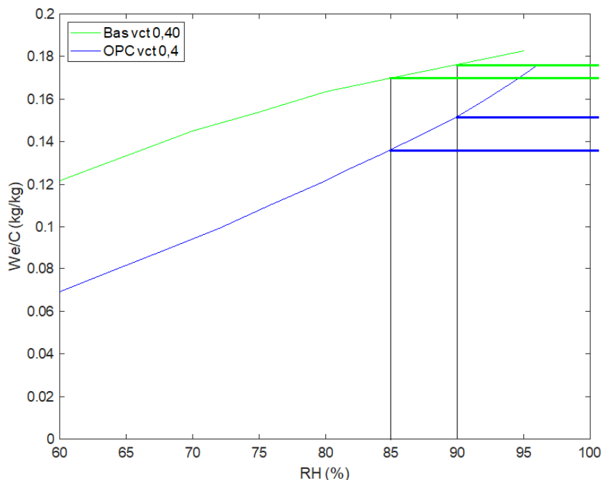
Figur 10. Fukthalt We/C som funktion av relativ fuktighet vid desorption för betong med Bascement (från Stelmarczyk m.fl. 2017b) resp. OPC (från Nilsson 1980), jämförelse av skillnad i fukthalt för skillnad i relativ fuktighet motsvarande 85% - 90%.
