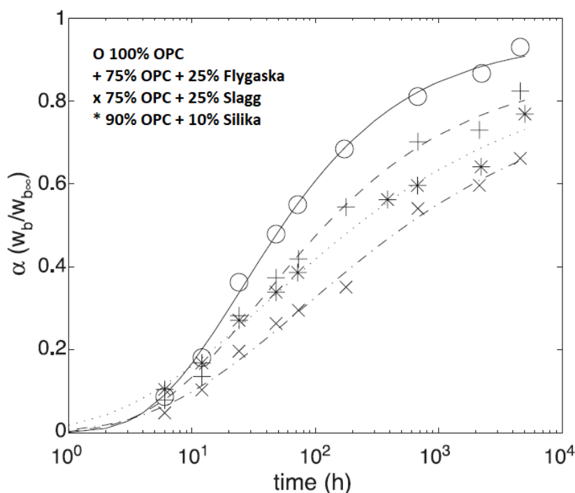
Figur 2. Hydratationsgrad \alpha , som funktion av tid, uppskattad från mängd kemiskt bundet vatten, för betong baserad på cement med olika bindemedelssammansättningar, härdad vid 23° C, från Pane & Hansen 2005.
