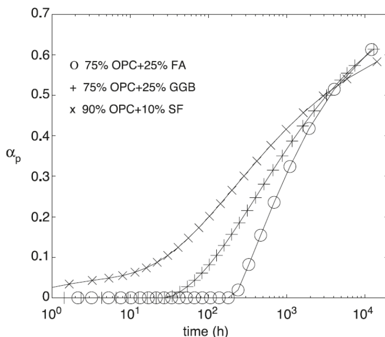
Figur 3. Reaktionsgrader \alpha_p , som funktioner av tid, för resp. tillsatsmaterial i blandningarna i Fig. 2, från Pane & Hansen 2005.
